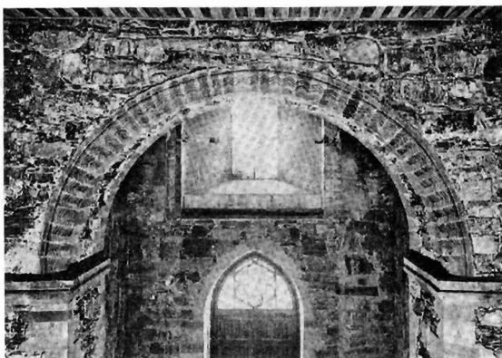
Den store buen bygd av romanske buesten. — The great arch, built of Romanesque voussoirs.
