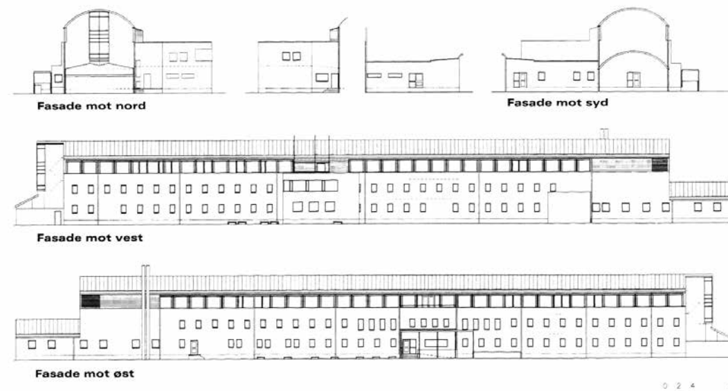
Fasadetegninger av Stavanger fengsel etter rehabiliteringen. Det nye taket skulle nedtone fengselsuttrykket. Foto: Statsbygg.
